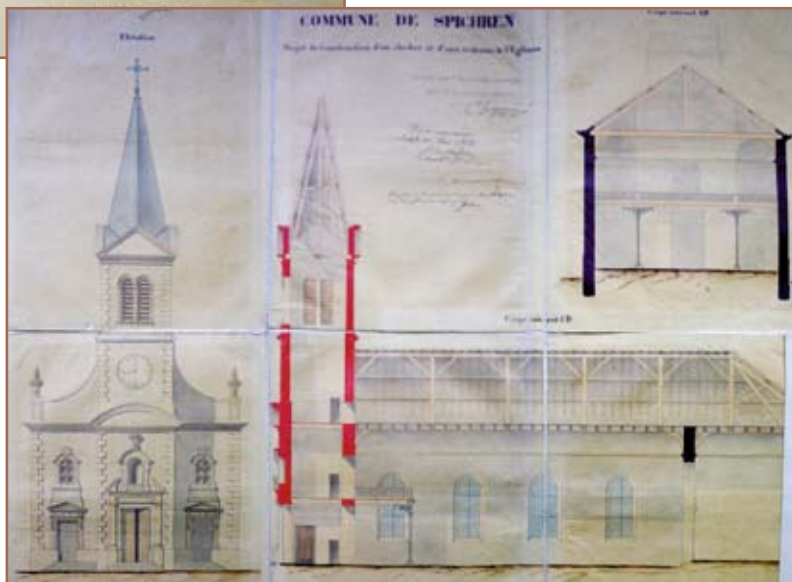
Projet de construction du nouveau clocher et de la tribune
